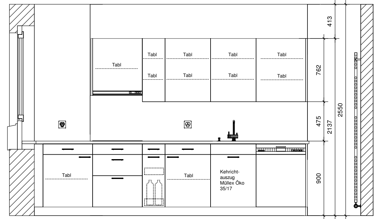
Ansicht A
