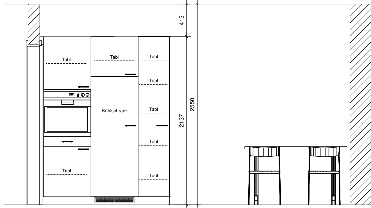
Ansicht B
